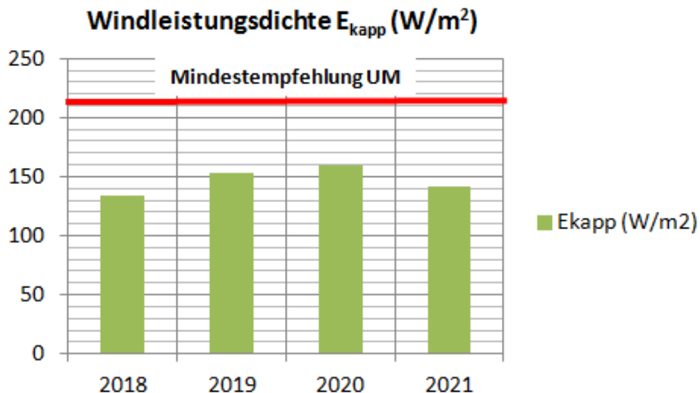
Abbildung 1: Mittlere gekappte Windleistungsdichte 2018 – 2021. Datenquelle: EnBW E-Cockpit, Darstellung: W. Fritz
